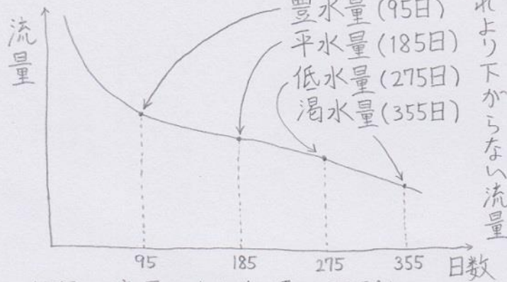
・流況曲線
